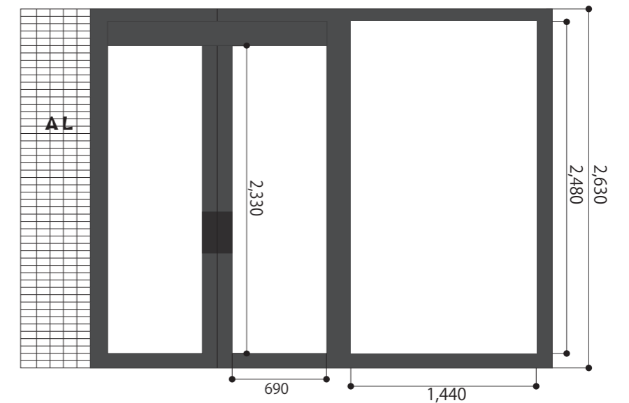
エントランスガラス寸法
